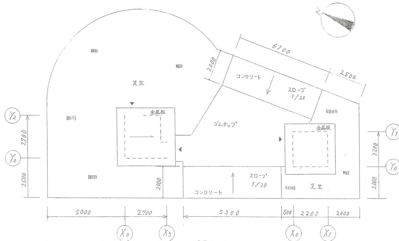
配置図 1/100
