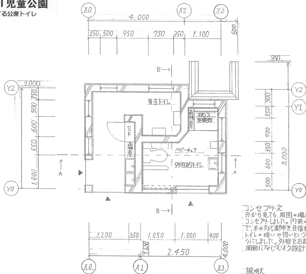
平面図 1:50
