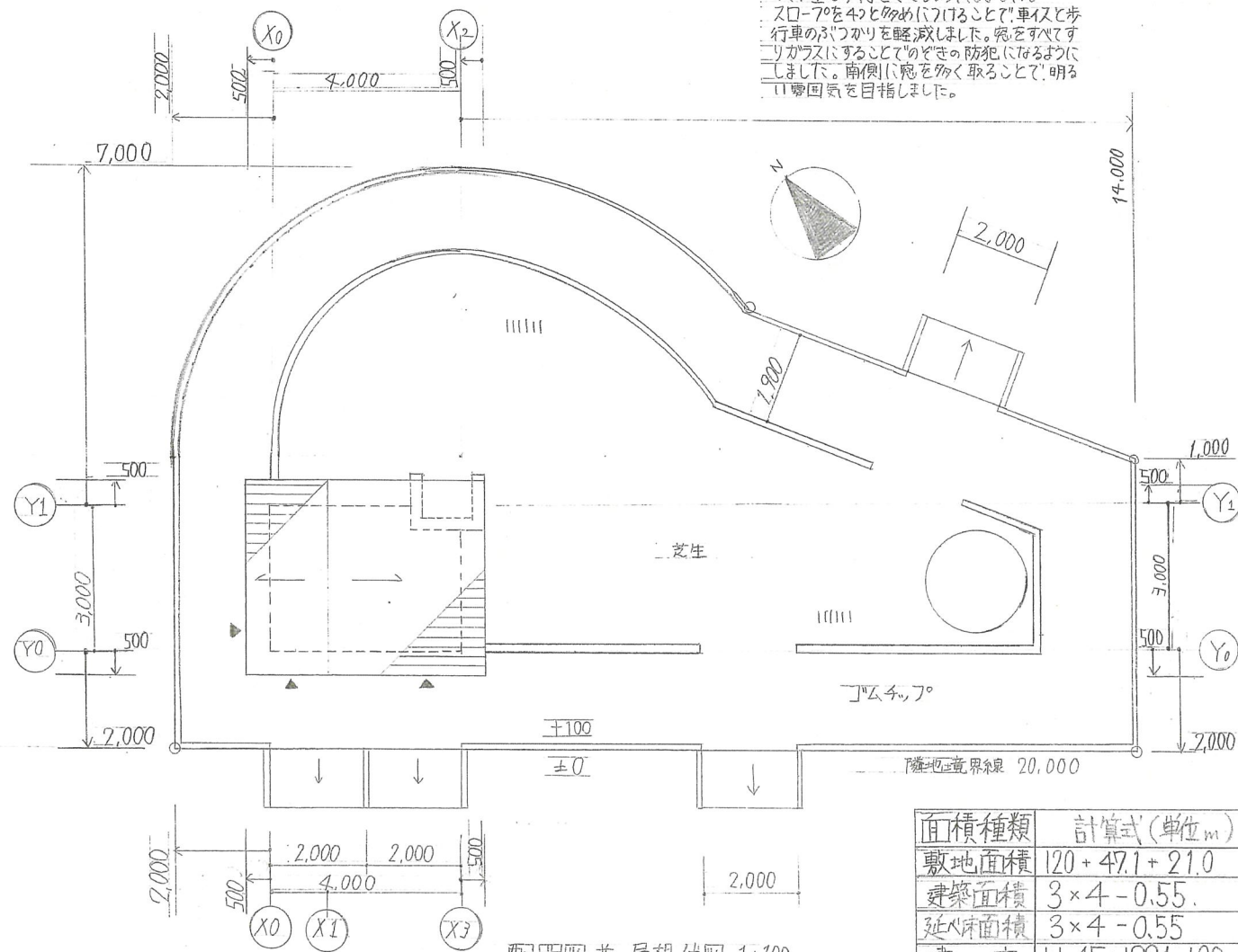
配置図兼屋根伏図 1:100
