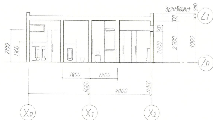
A-A断面図 1:100
