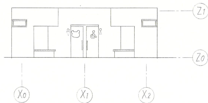
南立面図 1:100
