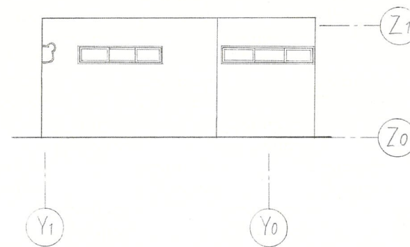
西立面図 1:100
