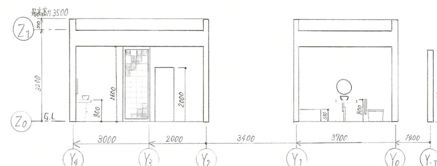
A-A断面図 1:100
