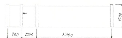
ドラッグラン立面図 1:100
