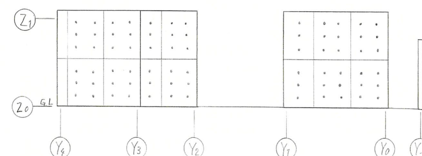
西立面図 1:100
