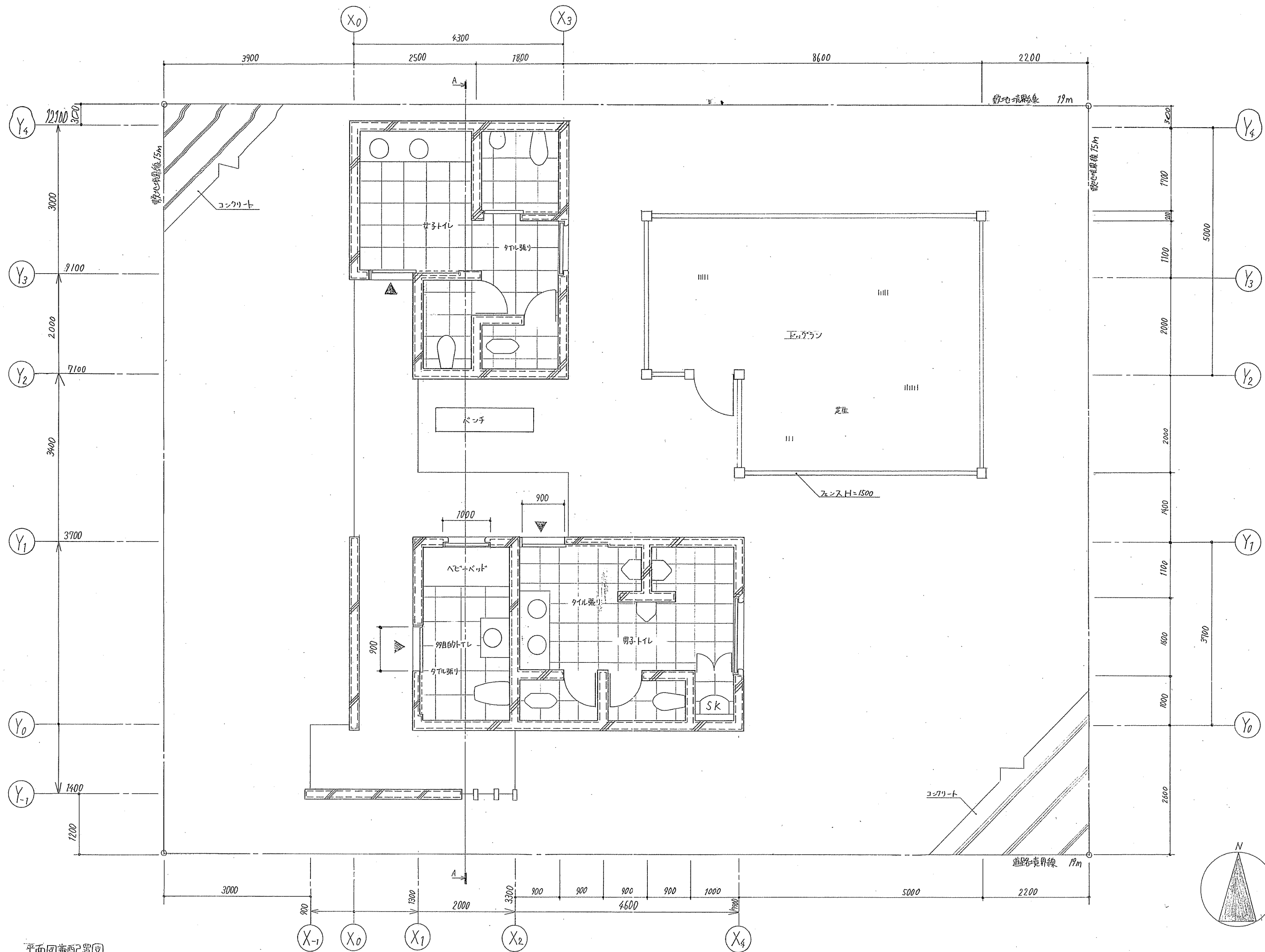
平面図兼西配置図 (1/50)
