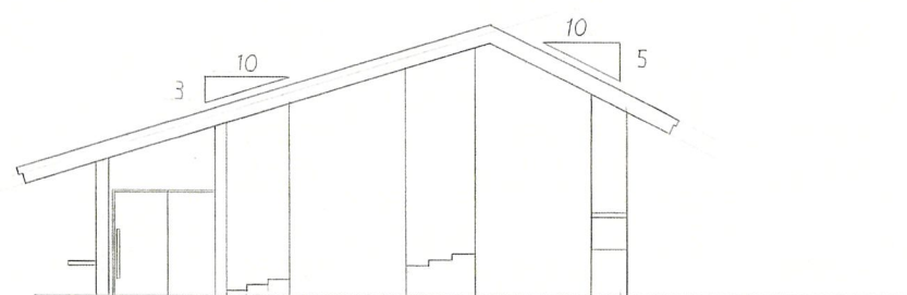
東立面図 1:100
