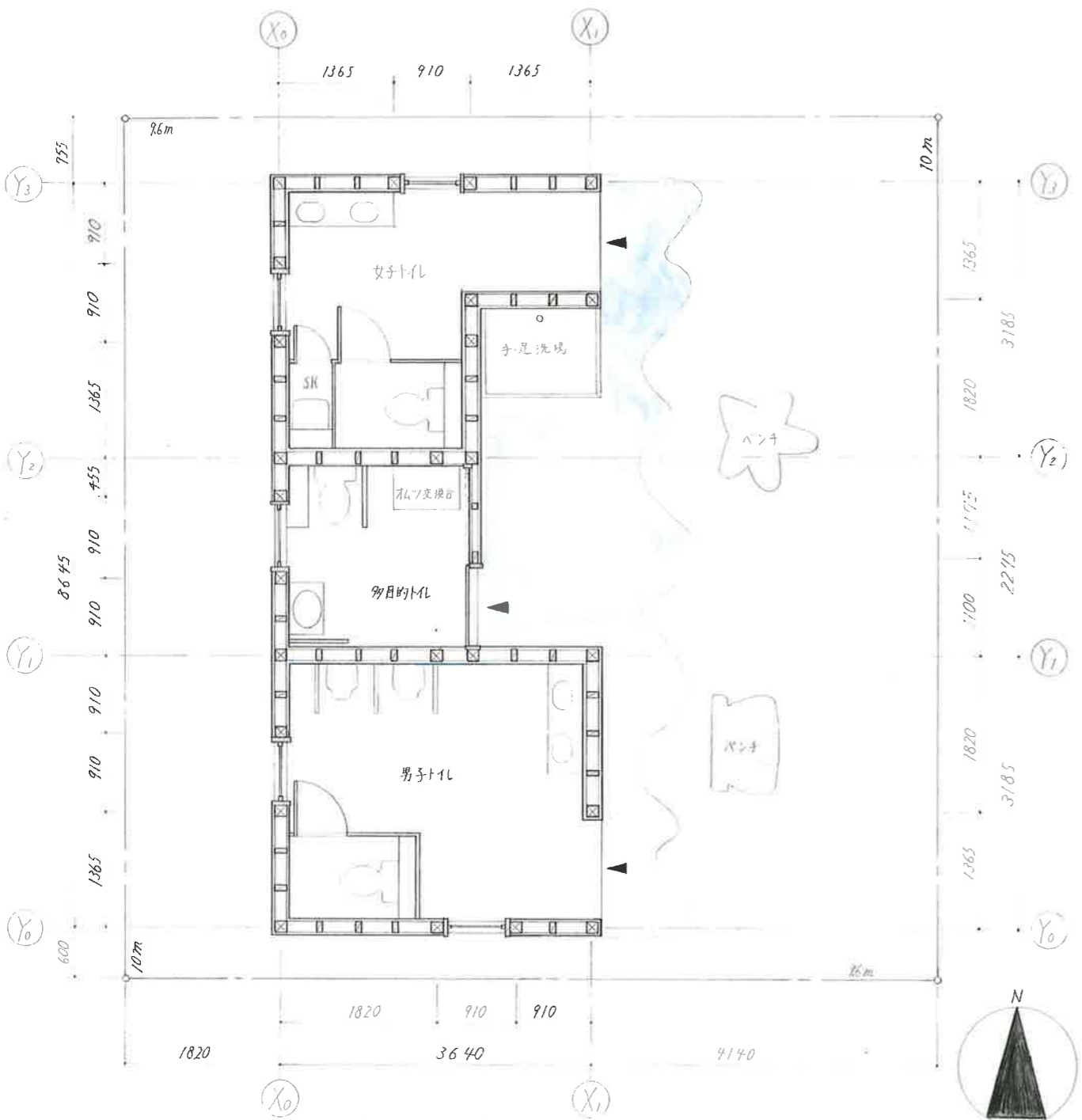
配置図 赤平図 1/50
