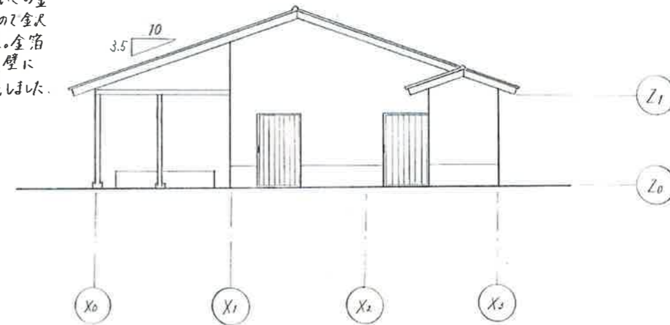
立面図 1:100
