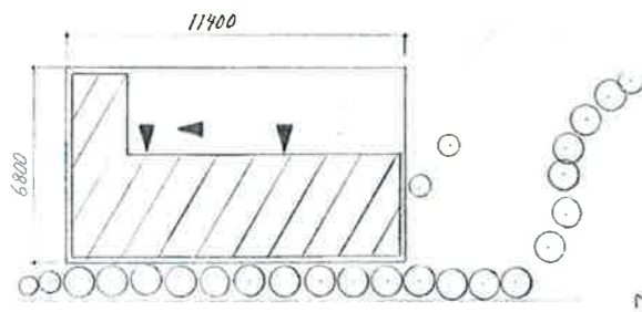
全体配置図 1:200
