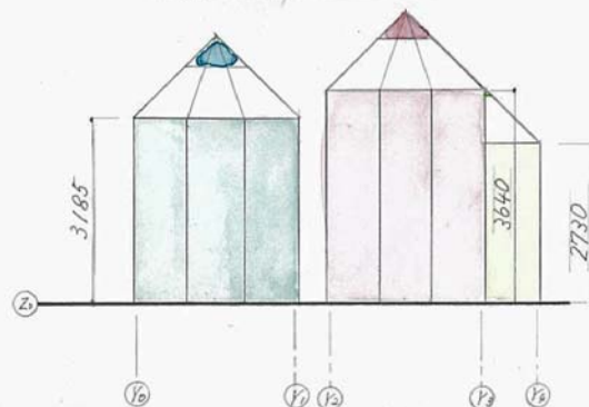
東立面圖 100:1
