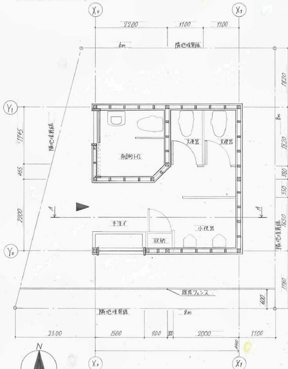
配置図兼平面図 1:50
