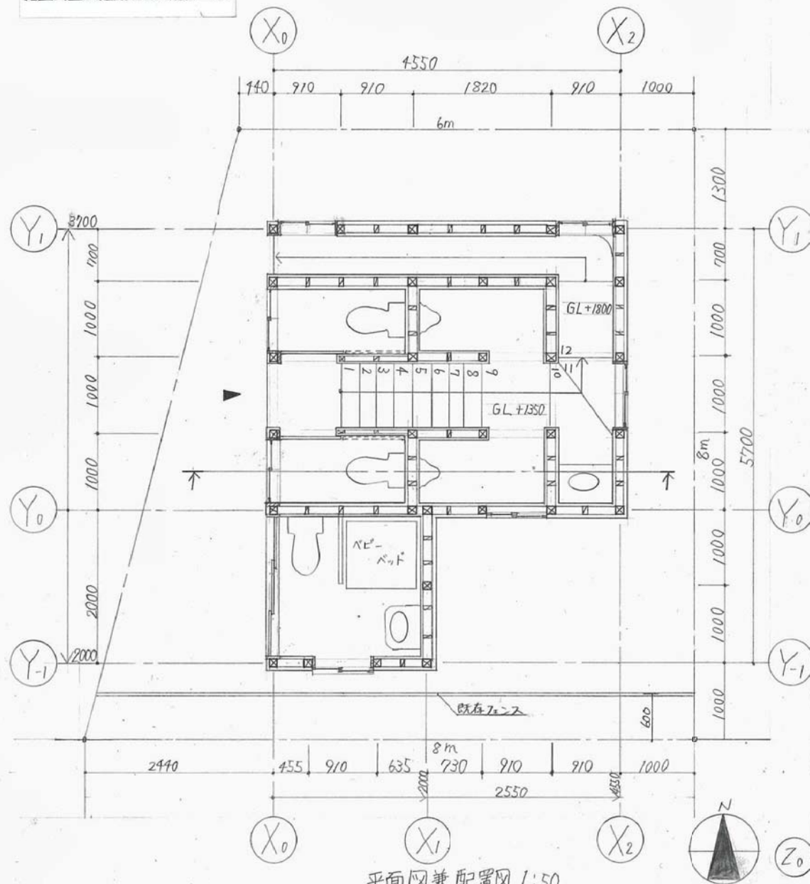
平面図兼配置図 1:50
