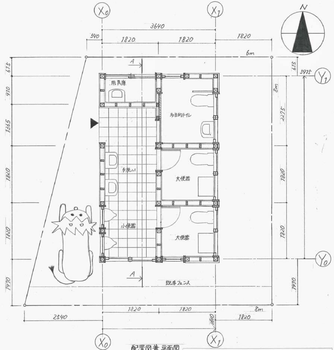
配置図兼平面図
