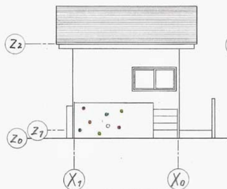
北立面图
