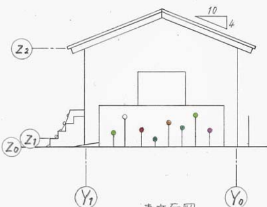
東立面圖
