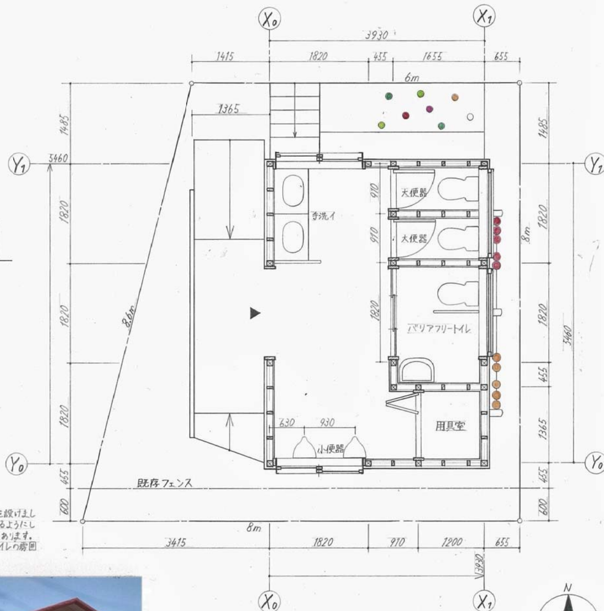
配置図兼平面図
