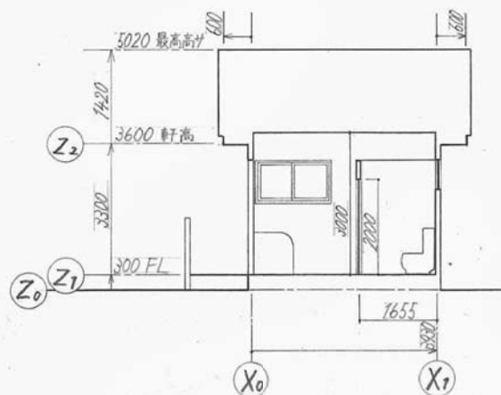
東立面圖
