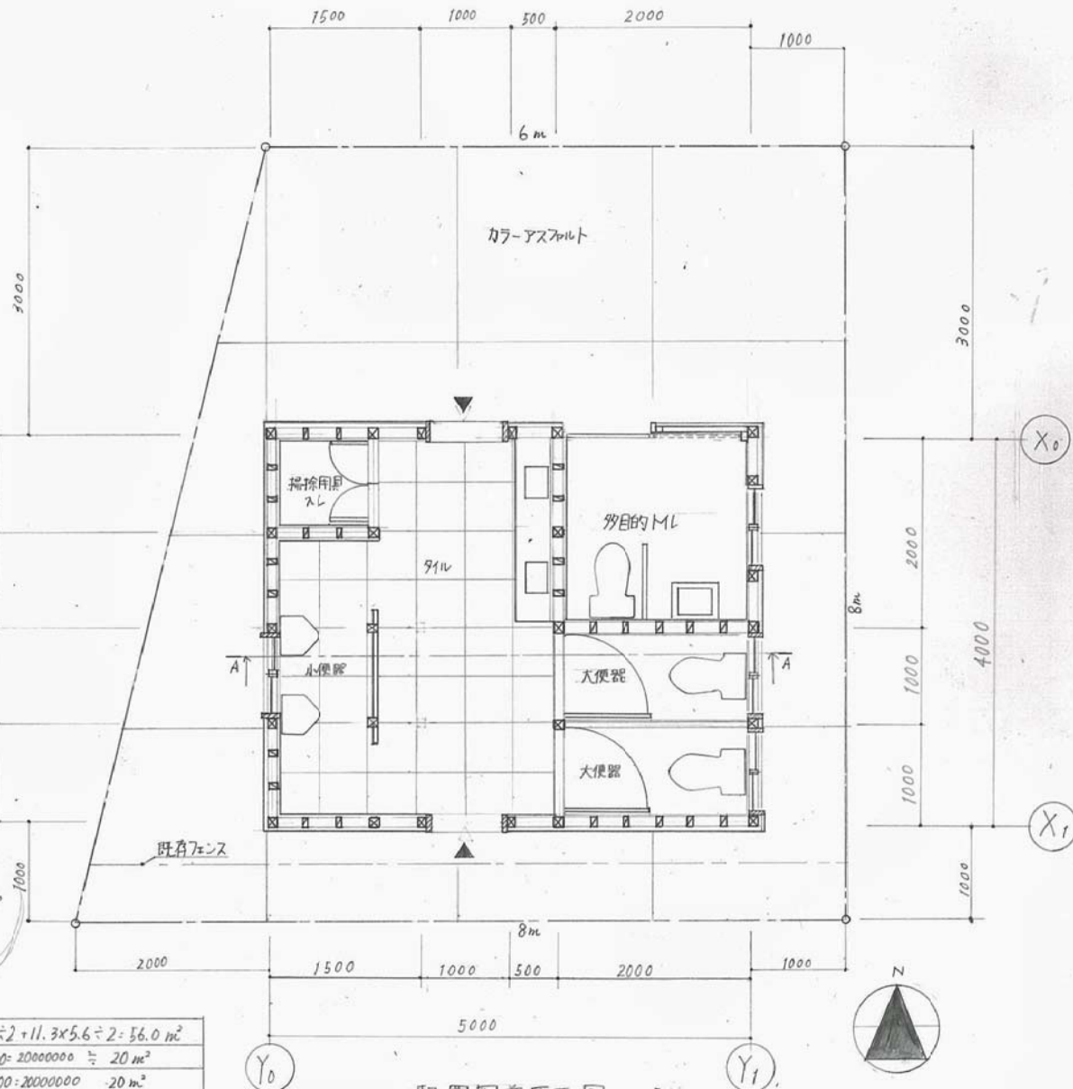
配置図兼平面図 1:50
