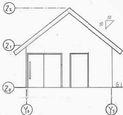
北立面图 1:100
