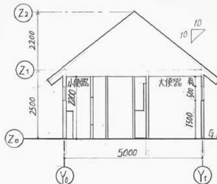
A-A 断面图 1:100
