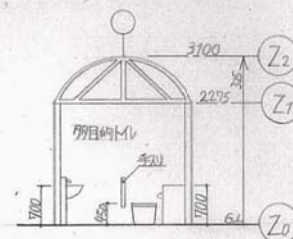
A-A断面図 1:100
