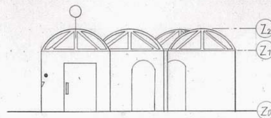
西立面図 1:100
