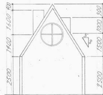
南立面図
