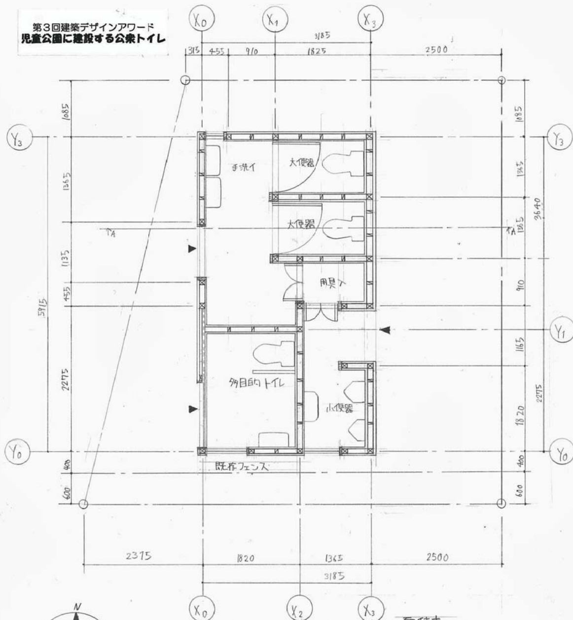
配置図兼平面図 1:50
