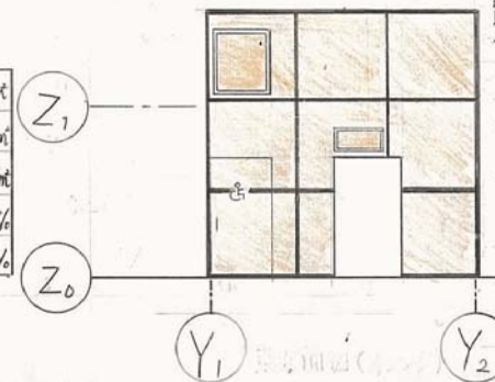
1/100 東立面図(オレンジ)
