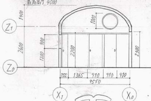
断面図 1/100
