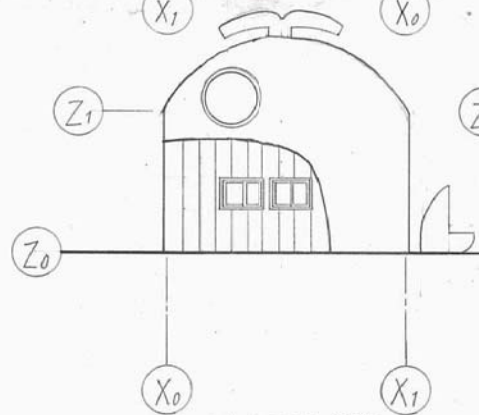
南立面図 1/100
