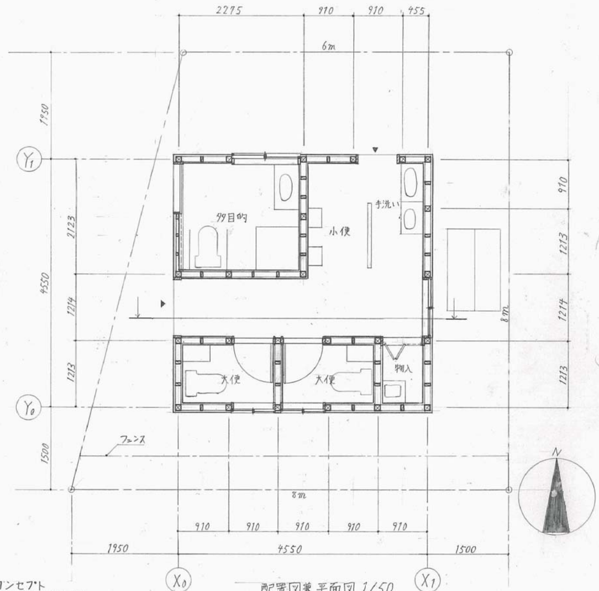
配置図兼平面図 1/50
