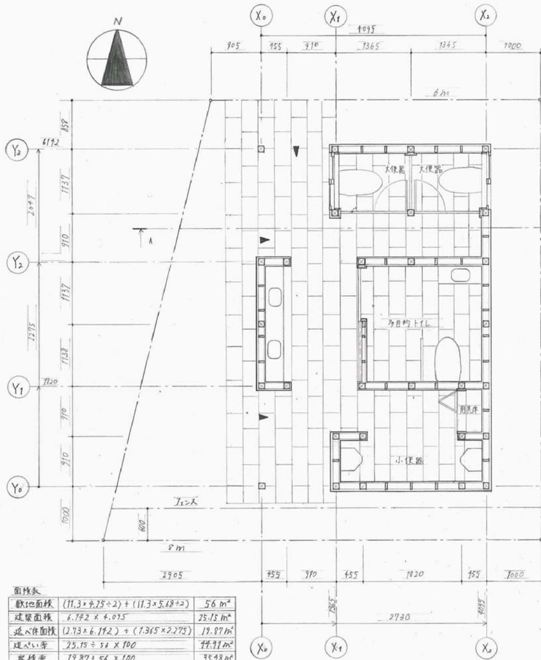
配置図兼平面図 1:50
