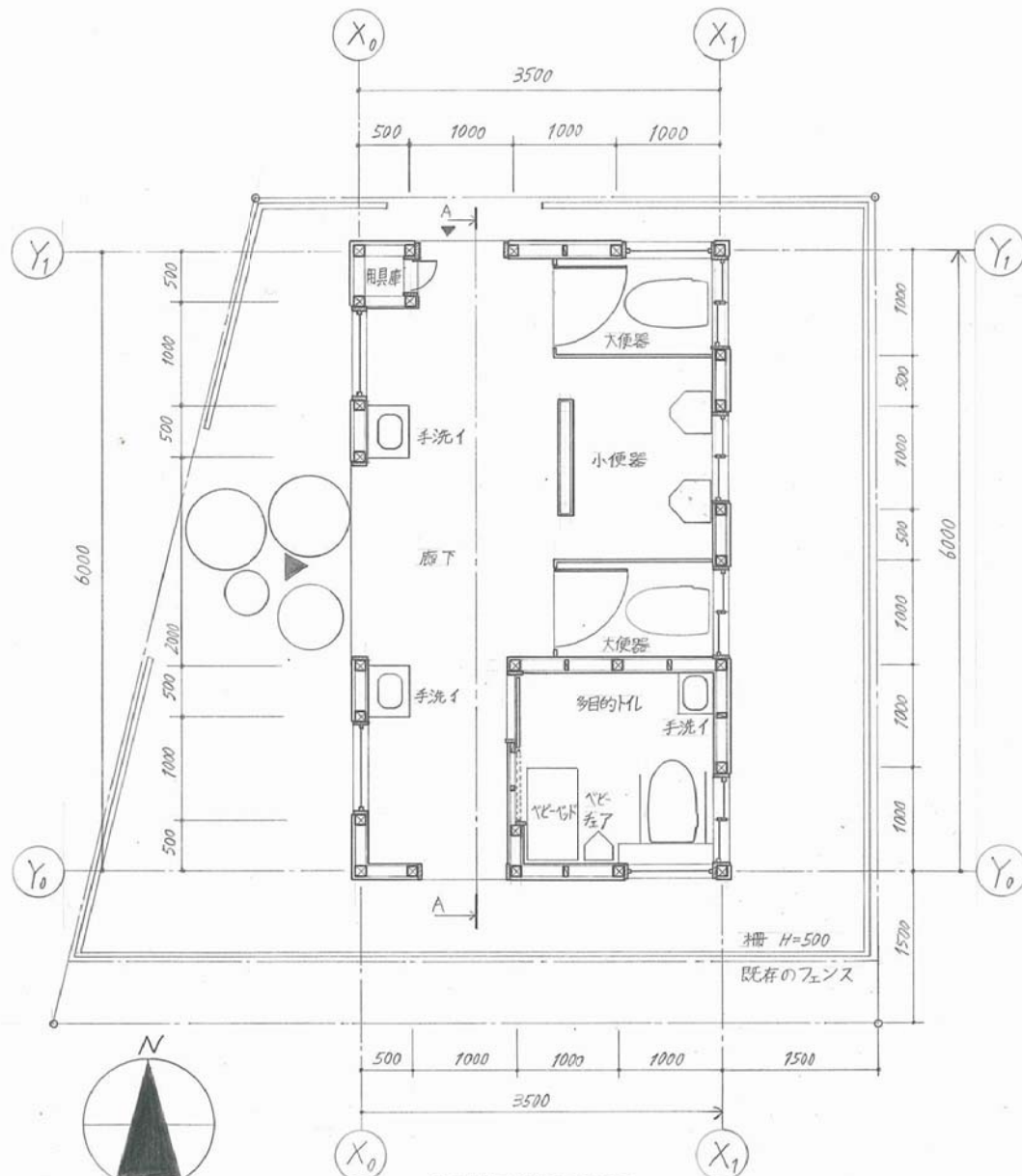
配置図兼平面図
