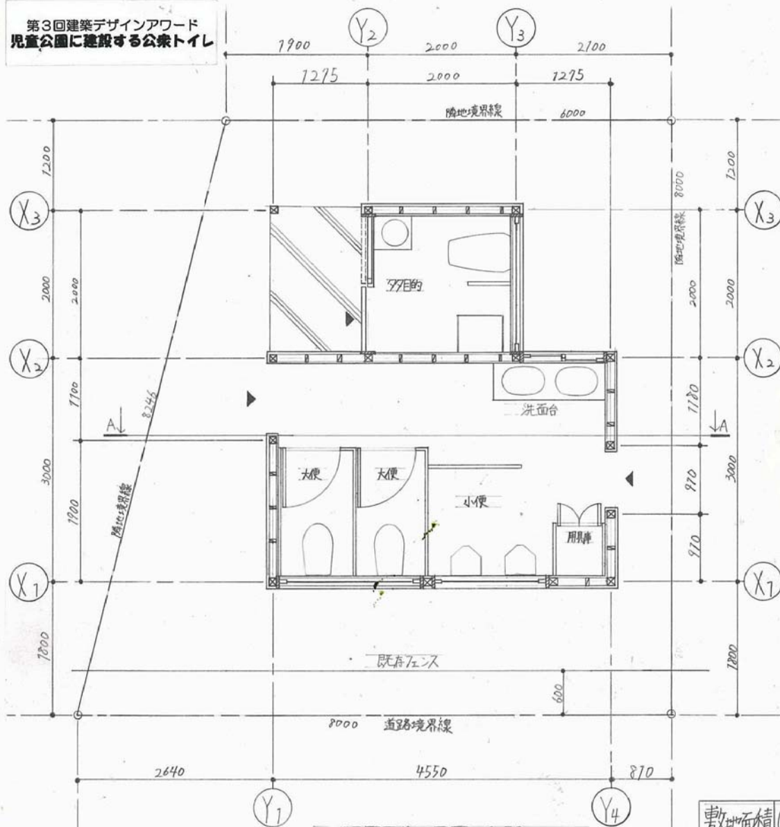
配置図兼平面図 1:50
