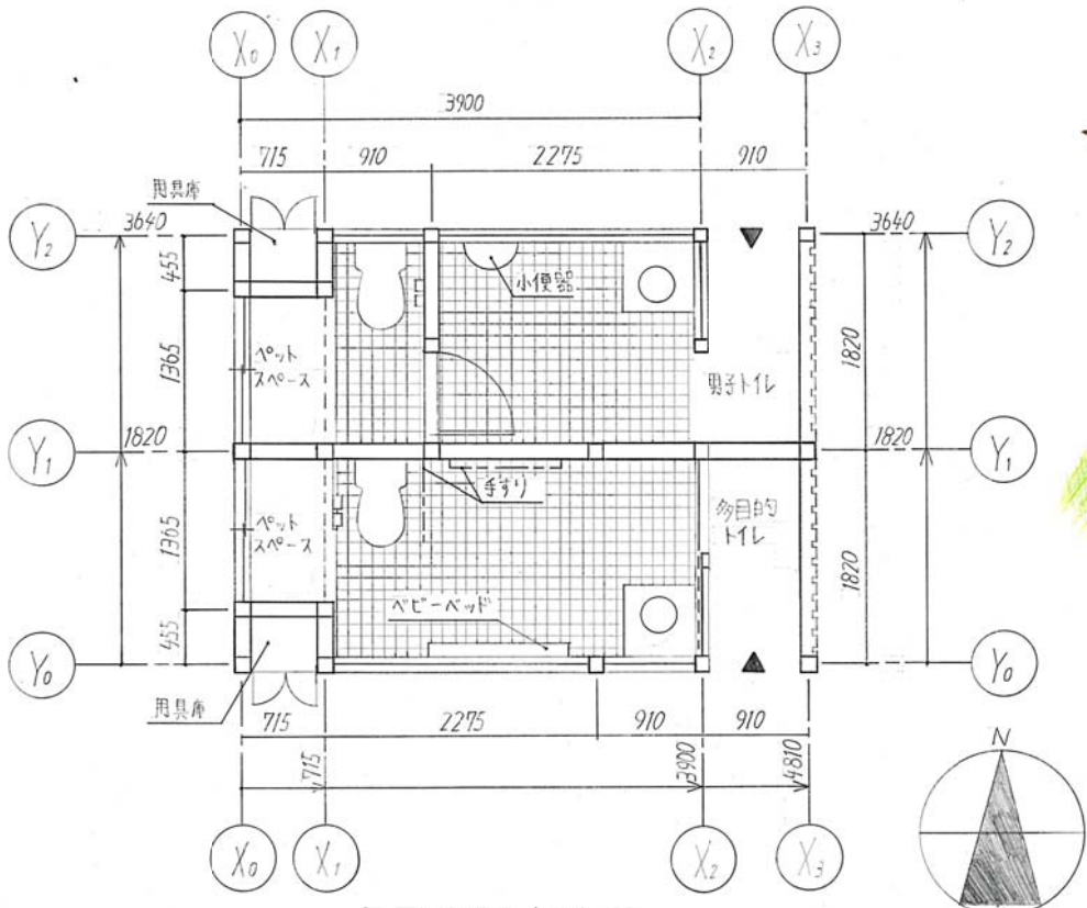
平面図 1:50
