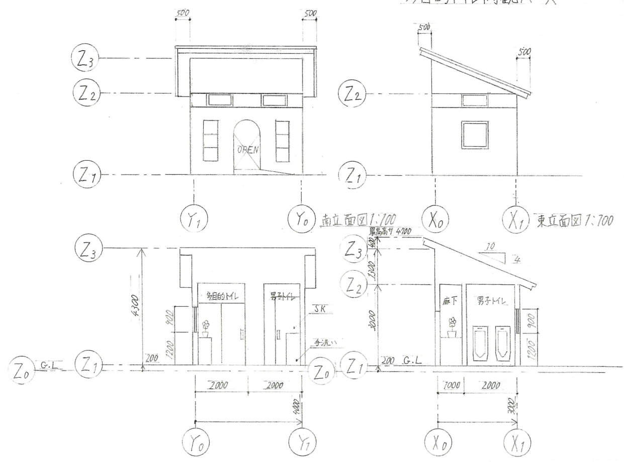
A-A断面図 1:100
