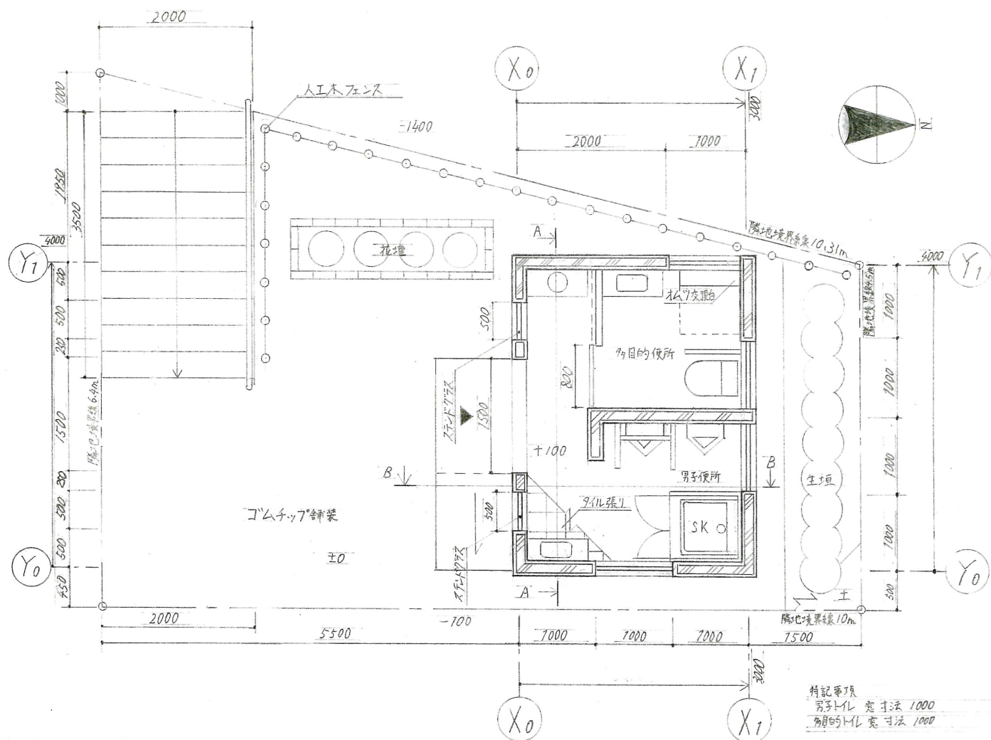
配置図兼平面図 1:50
