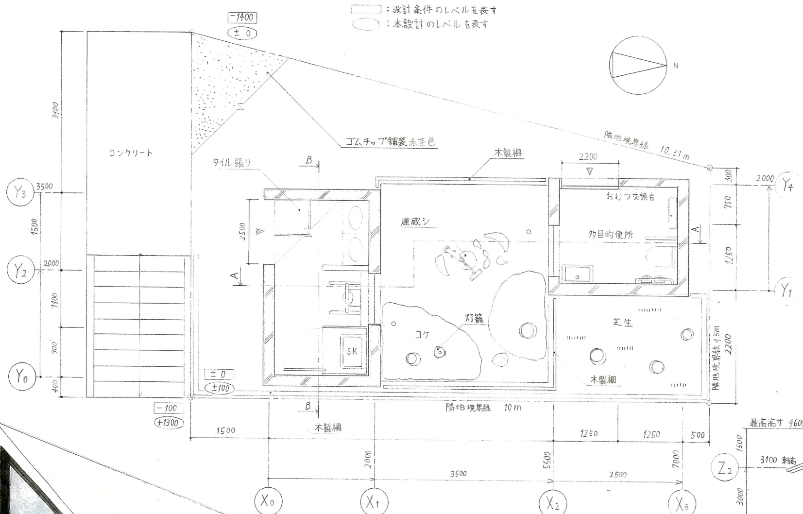
配置図兼平面図 1:50
