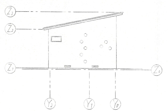
南立面図 1/100
