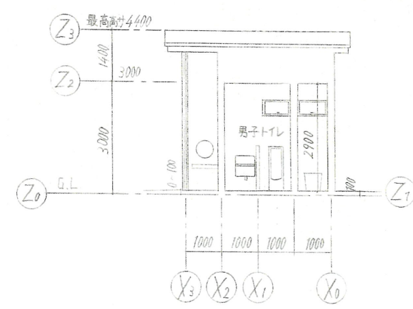
北立面図 1/100
