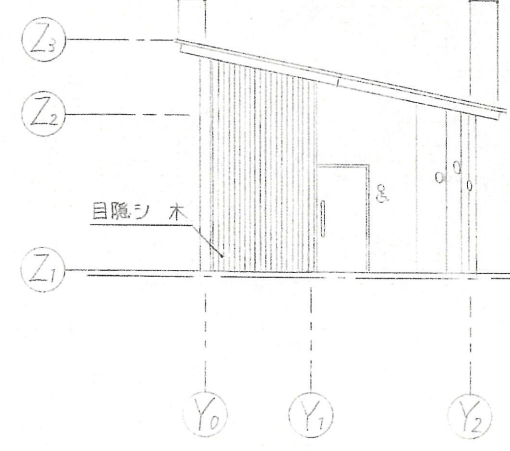
北立面図 1/100
