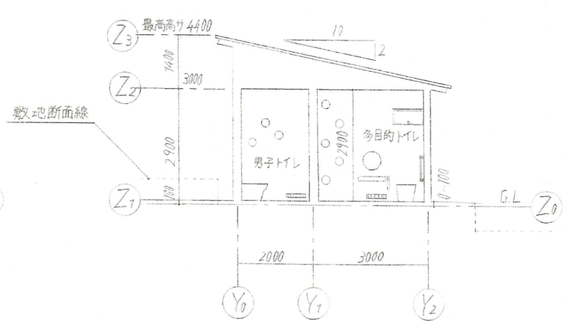
B-B断面図 1/100
