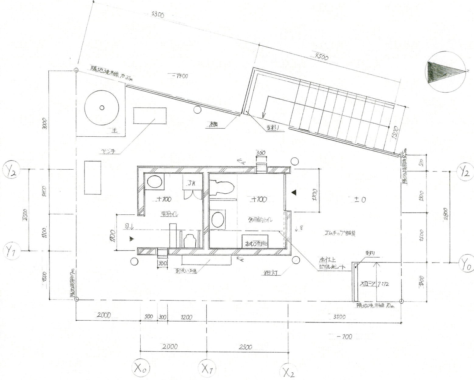
配置図兼平面図 7:50
