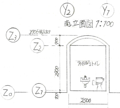
A-A断面図 7:700
