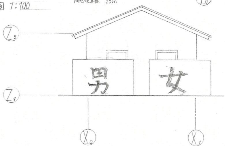
南西立面図 1:100
