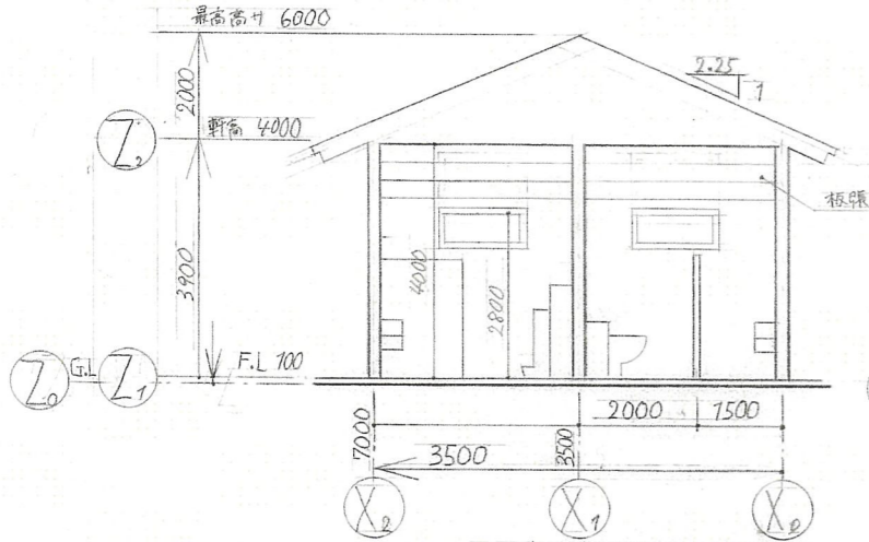
A-A断面図 1:100
