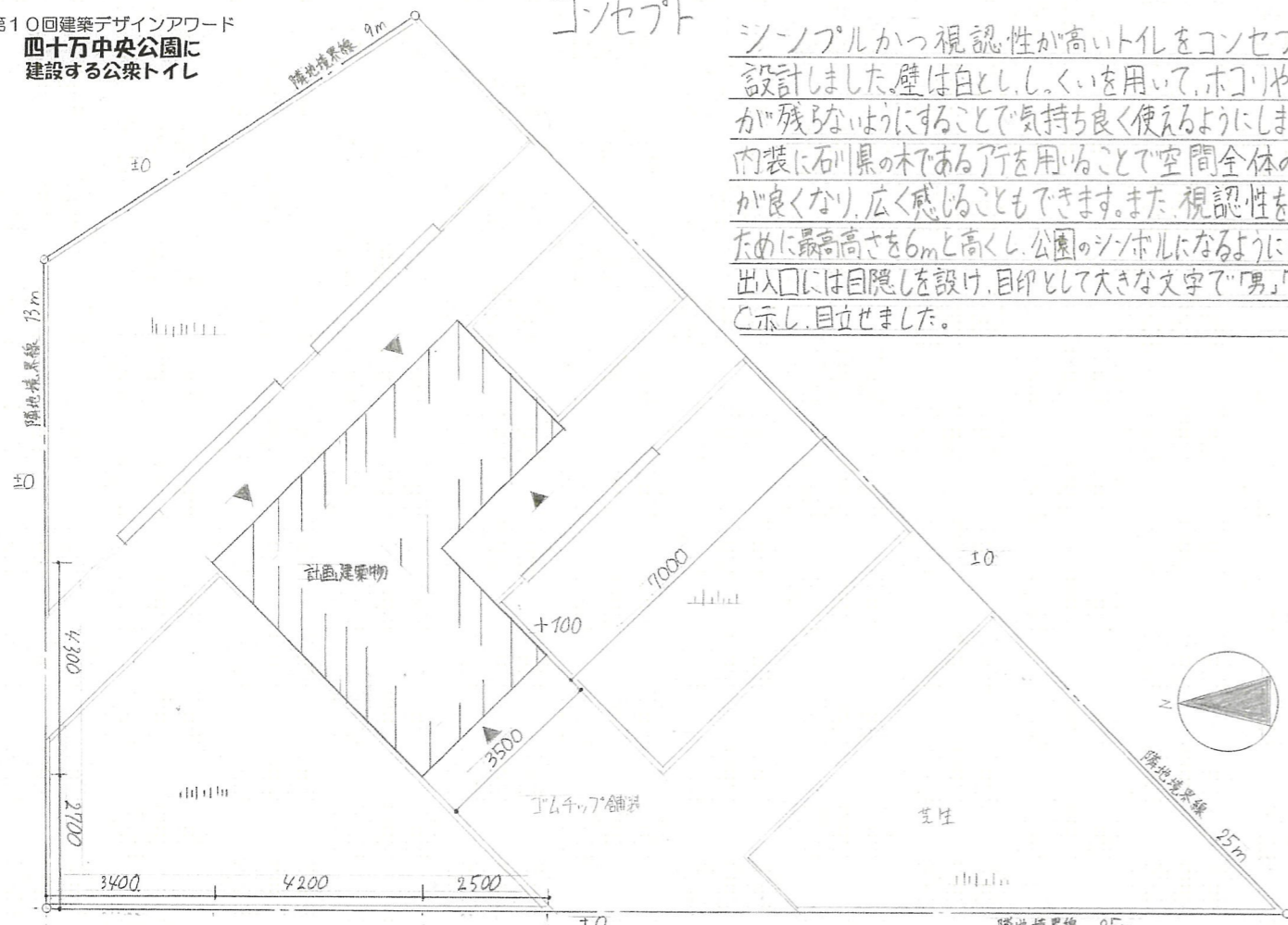
全体配置図 1:100
