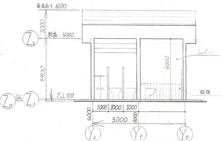
B-B断面図 1:100
