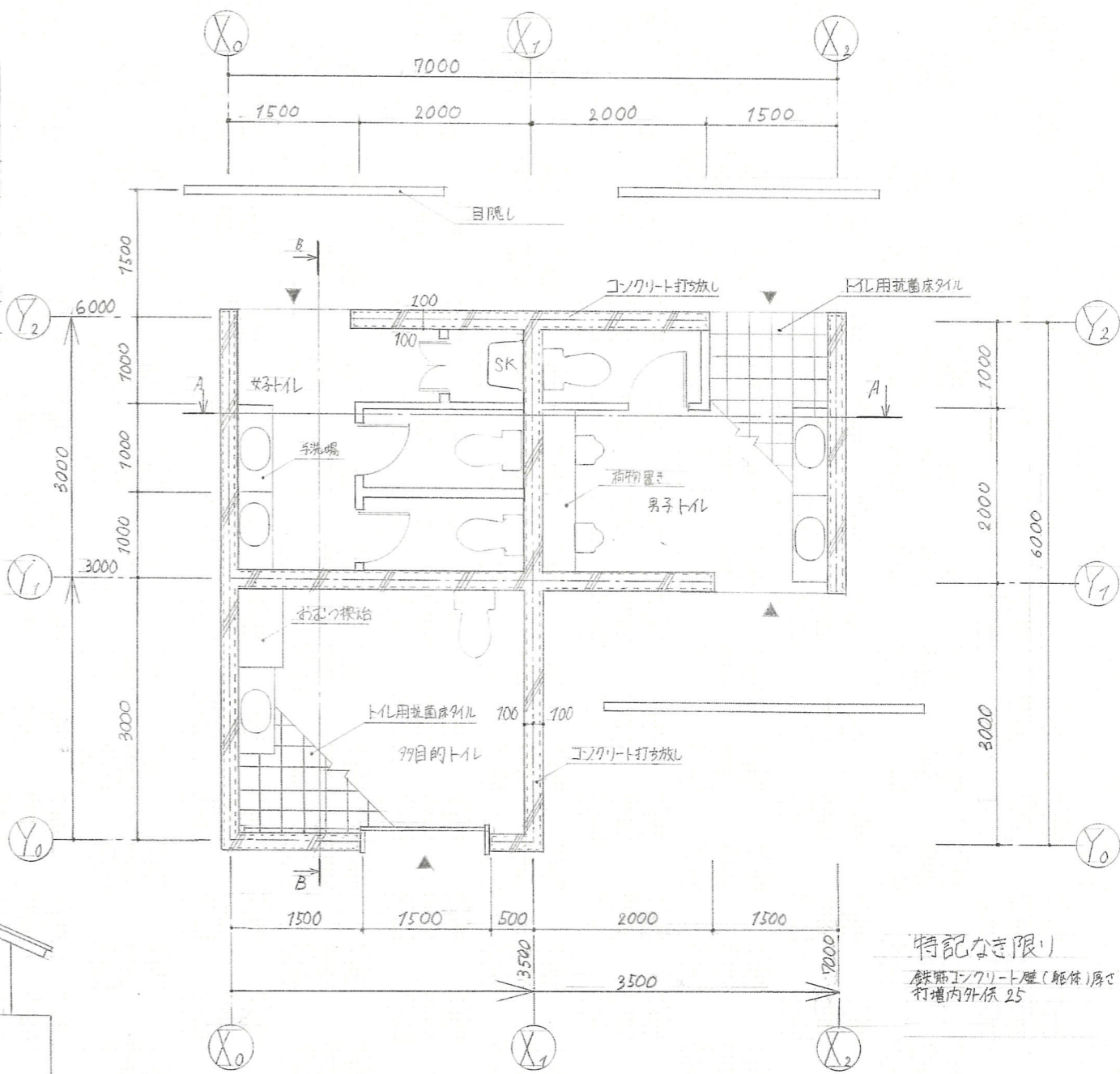
平面図 1:50
