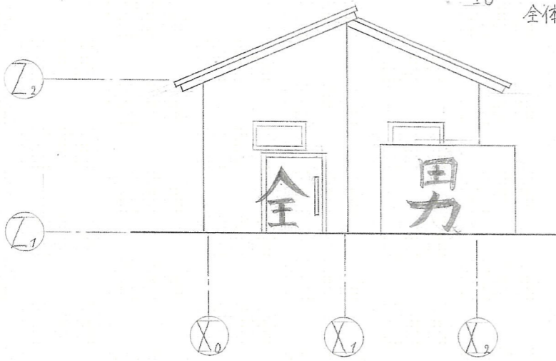
北東立面図 1:100
