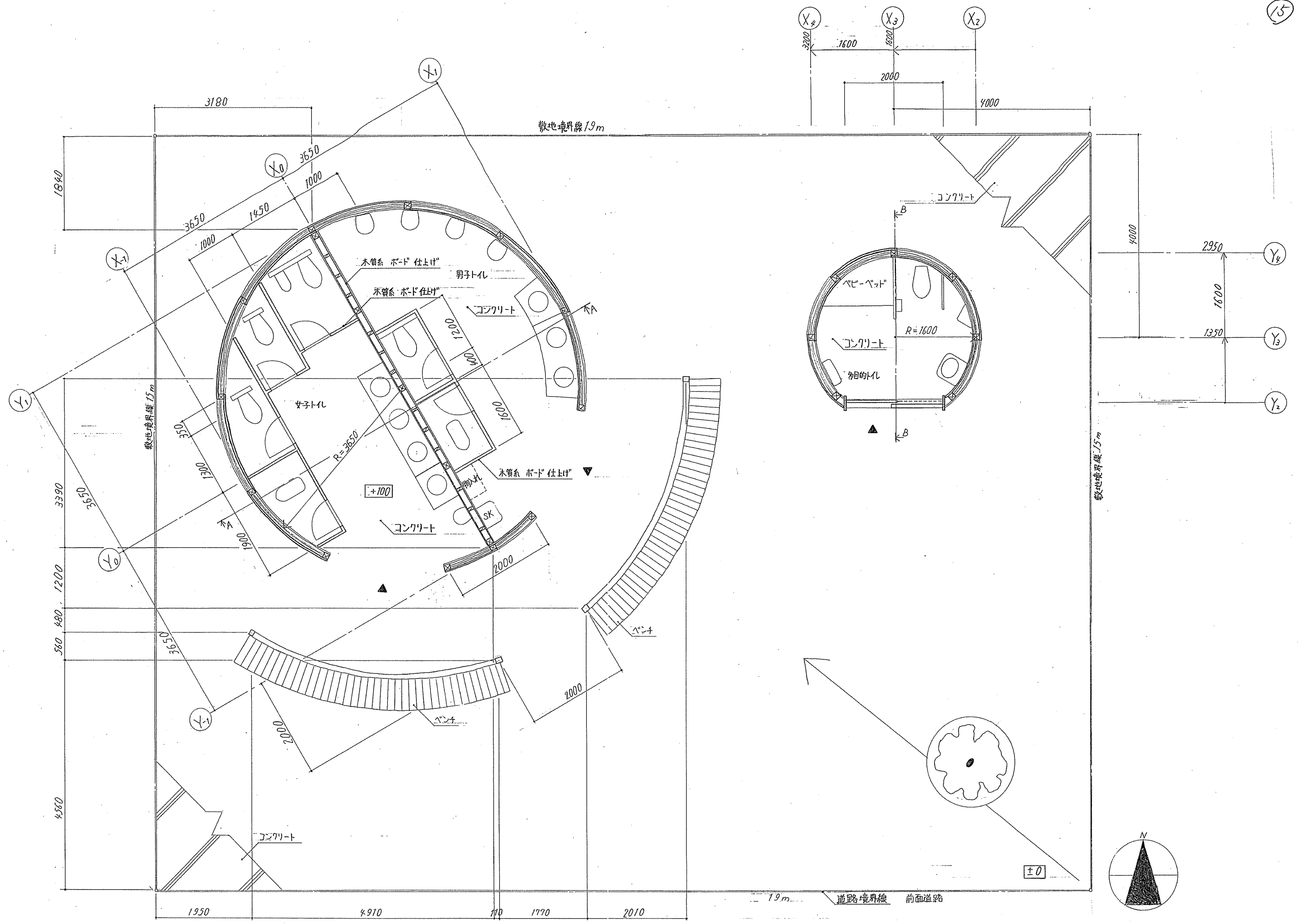
平面図兼配置図 1:50
