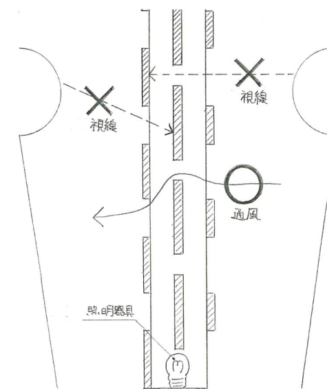
外壁の構成
