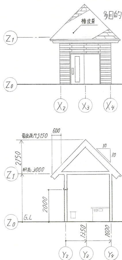
B-B断面図 1:100
