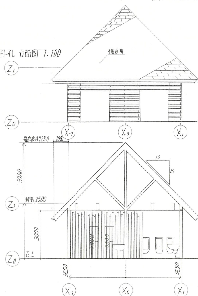
A-A断面図 1:100
