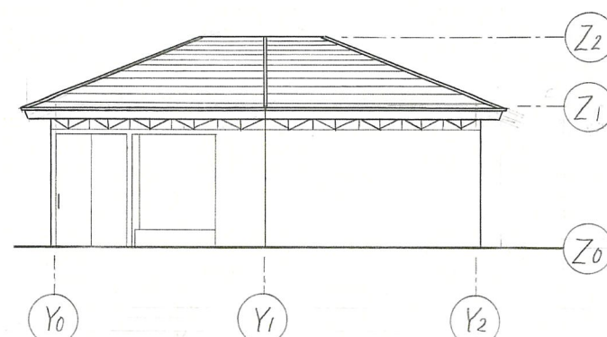
東立面図 1:100
