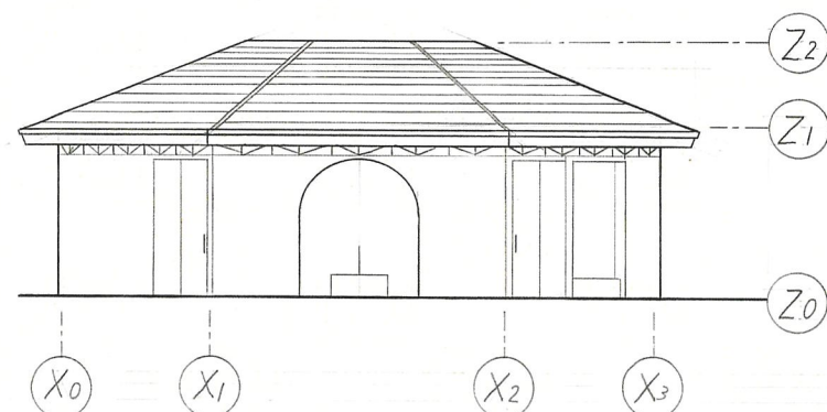
南立面図 1:100
