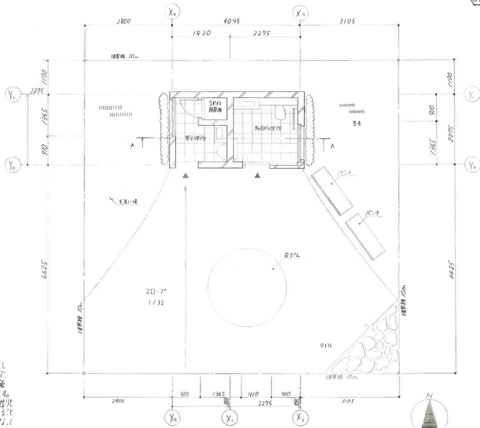
西配置兼平面図 1:50
