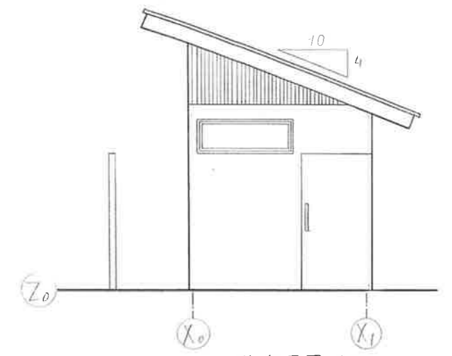
北立面図 1:50
