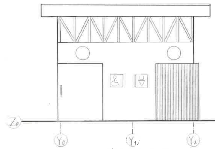
東立面図 1:50
