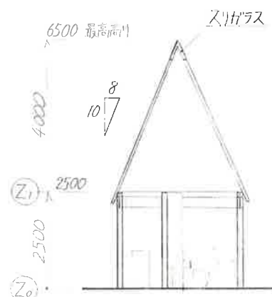
A-A 断面図
