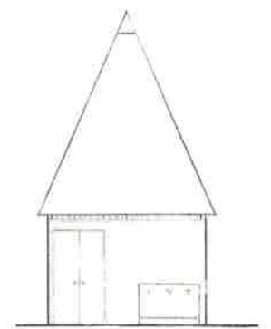
東立面図
