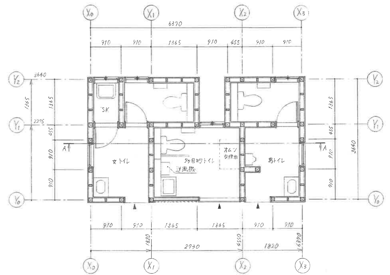
平面図 1:50
