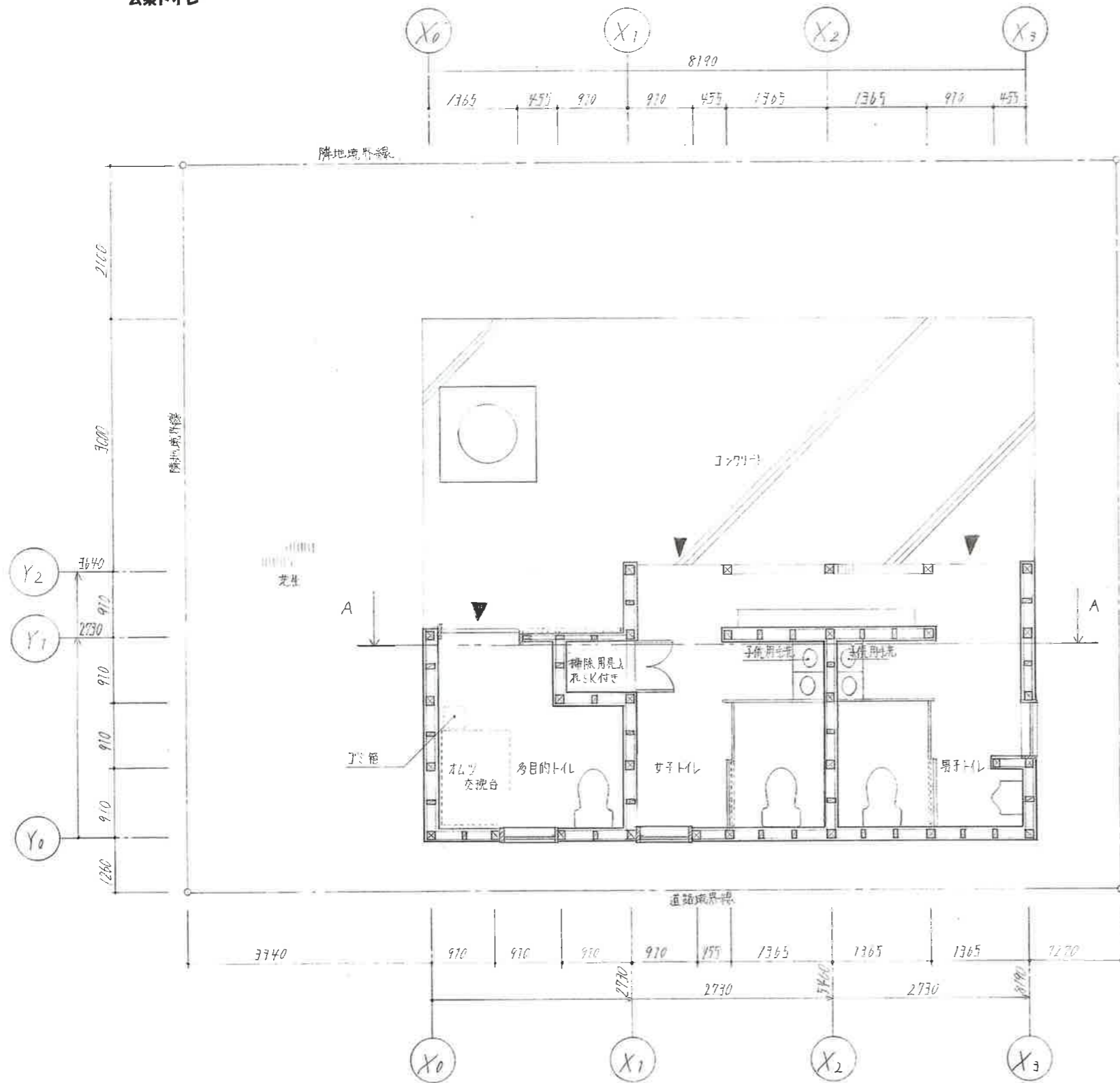
配置図 兼 1階平面図 1:50
