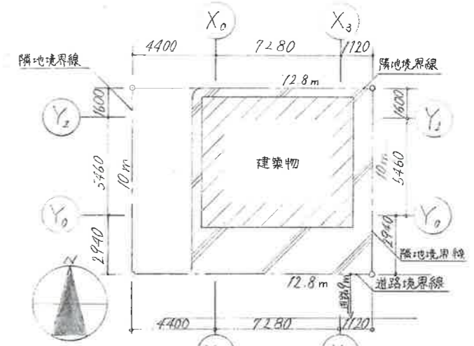
配置図 1:200
