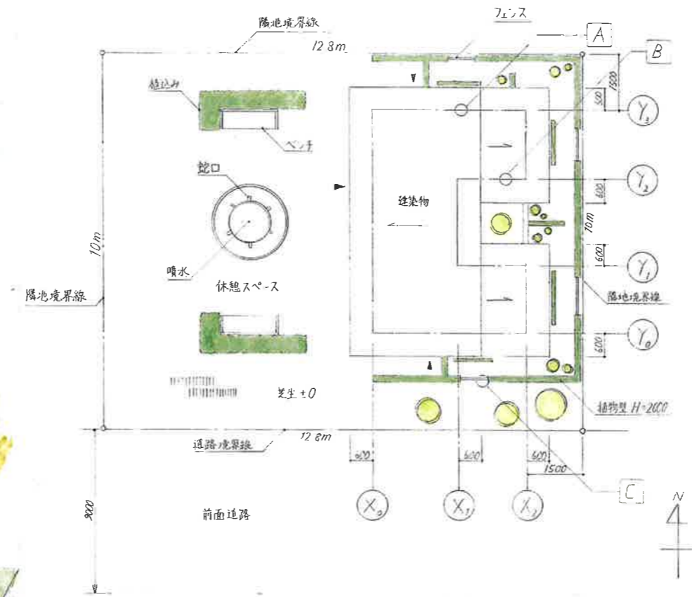
配置図兼屋根伏図 1:100
