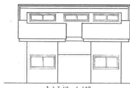
東立面図 1:100
