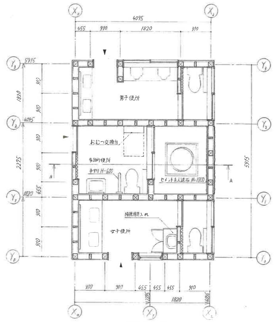
平面図 1:50
