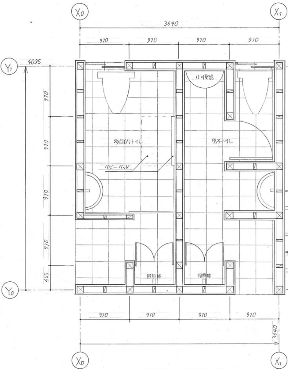
平面図 尺度 1:30
