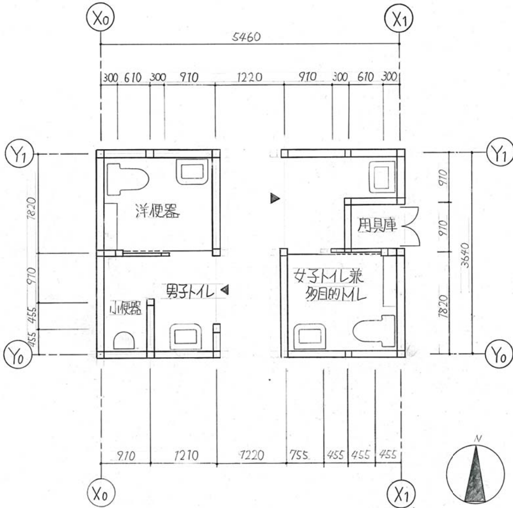
平面図 1:50
