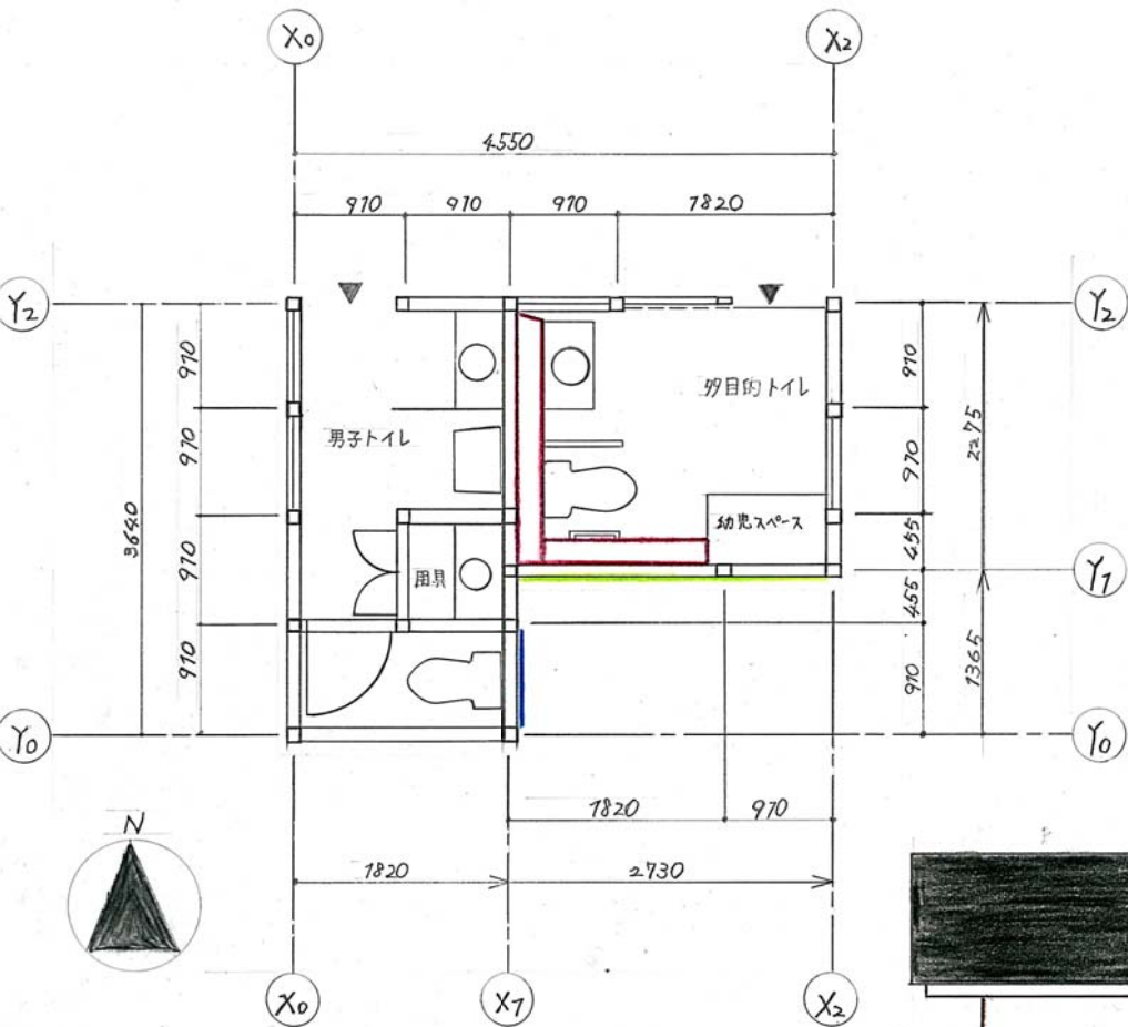
平面図 1:50
