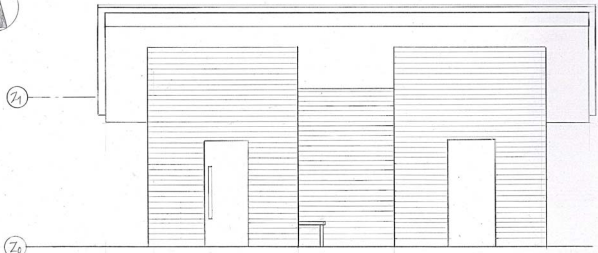
南立面図
