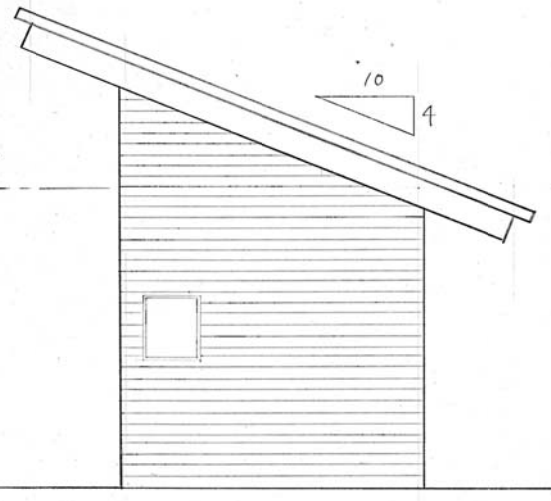
東立面図
